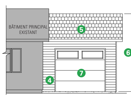
8 ÉLÉVATION AVANT
