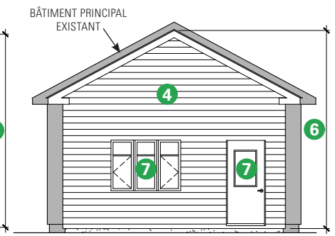
8 ÉLÉVATION LATÉRALE
