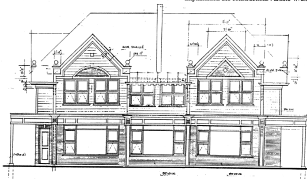
COMMERCE ÉLEVATION PRINCIPALE / RUE JEAN-JUNEAU ÉCHELLE : 1/8" = 1'-0"
