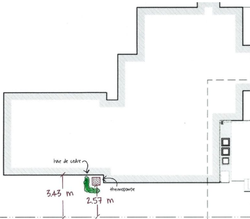
Plan de la position souhaitée de la thermopompe
