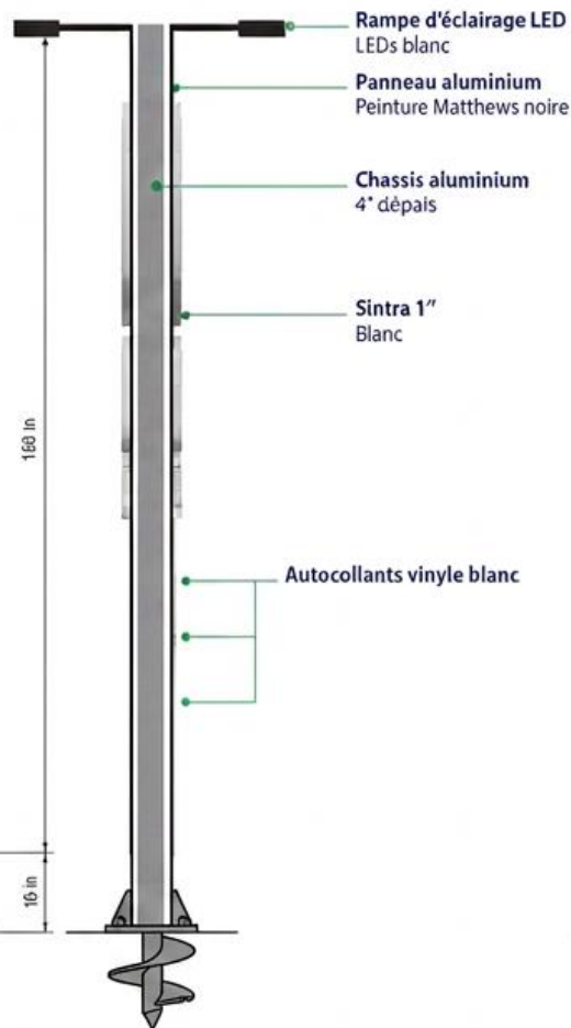
VUE LATÉRALE
